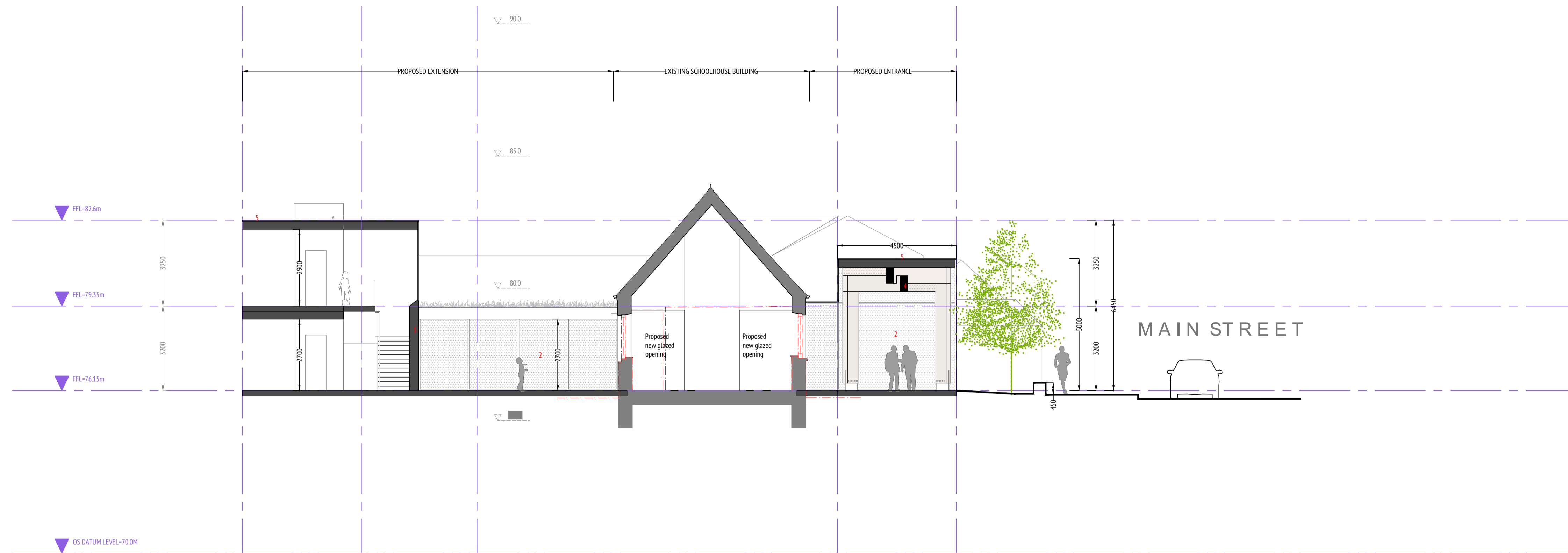
SECTION A-A
